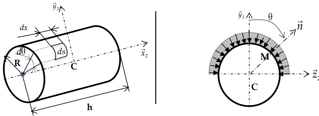
Figure 11 : Modèle retenu et paramétrage
