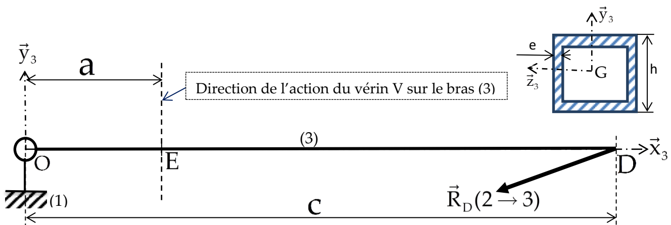
Figure13 : Le modèle poutre retenu pour le bras (3)
