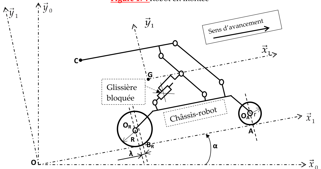
Figure 17 : Robot en montée
