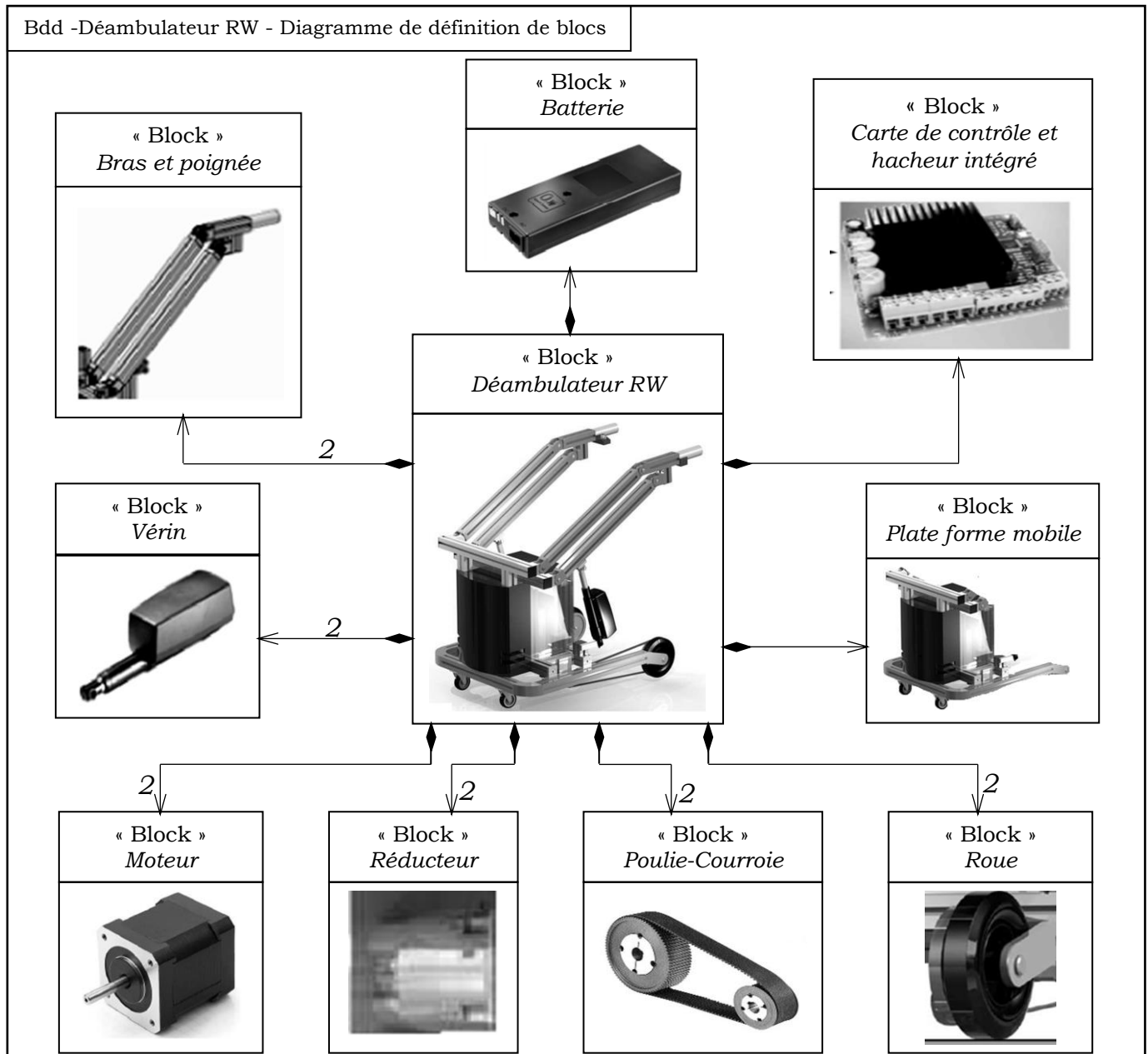
Figure 6 : Diagramme de définition de blocs partiel
