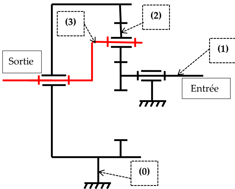
Figure 16 : Désignation du réducteur épicycloïdal
