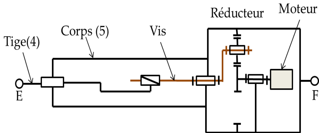
Figure15 : Vérin électrique
