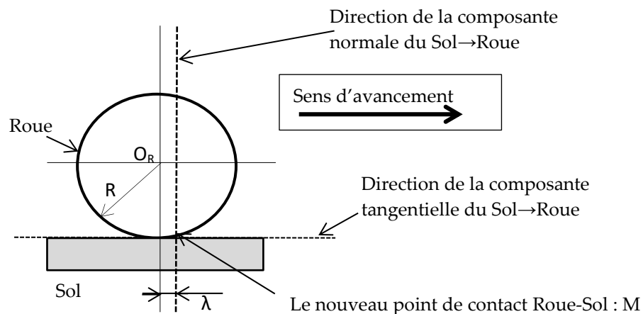
Figure 18 : Modèle résistance au roulement
