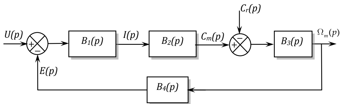
Figure 11 : schéma fonctionnel du moteur
