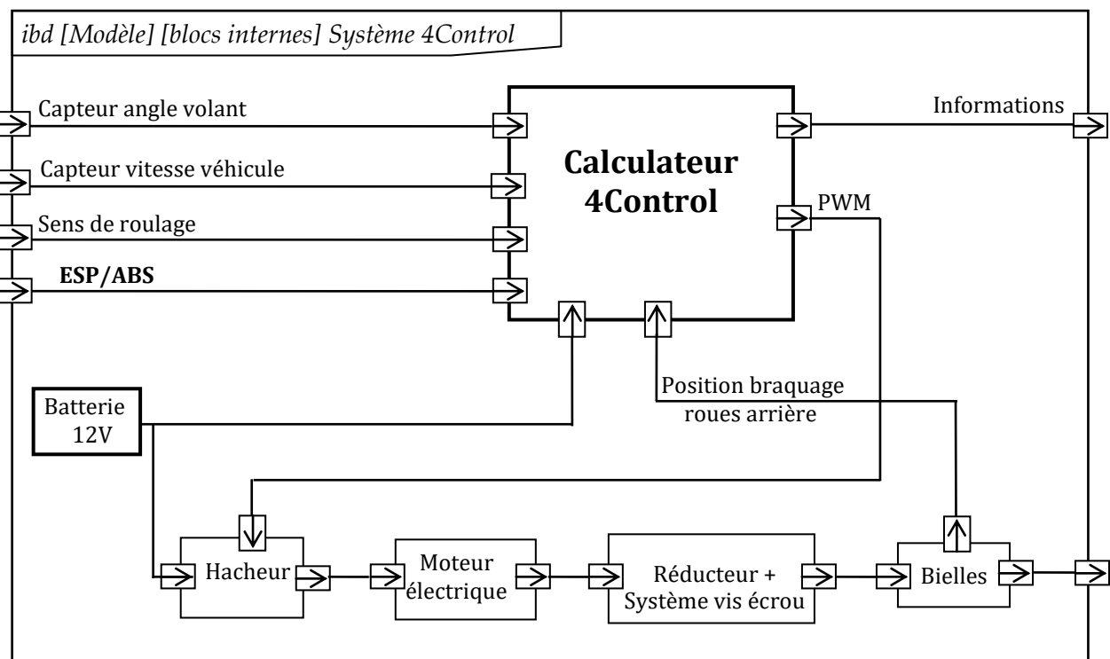
Diagramme des blocs internes du système 4Control
