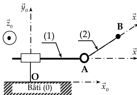
Figure 3 : Schéma cinématique partiel.
