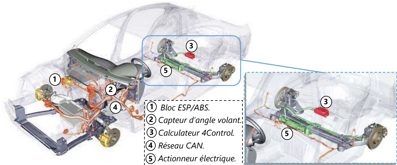
Figure 2 : Système 4Control (RENAULT)
