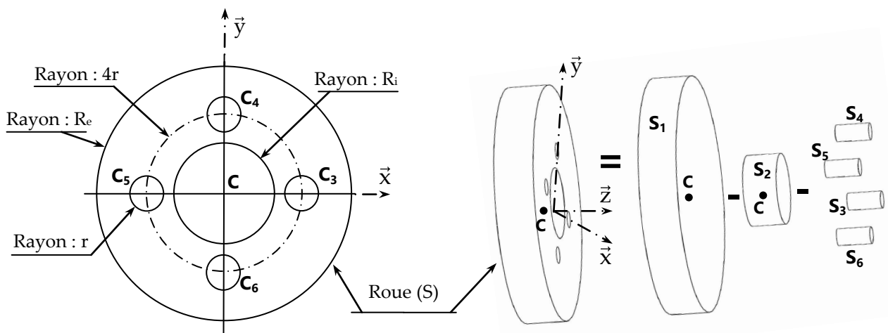
Figure 4 : modèle géométrique simplifié de la roue.
