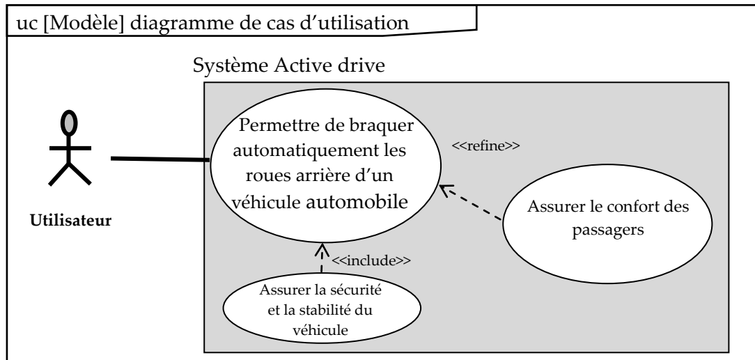
Diagramme de cas d'utilisation.
