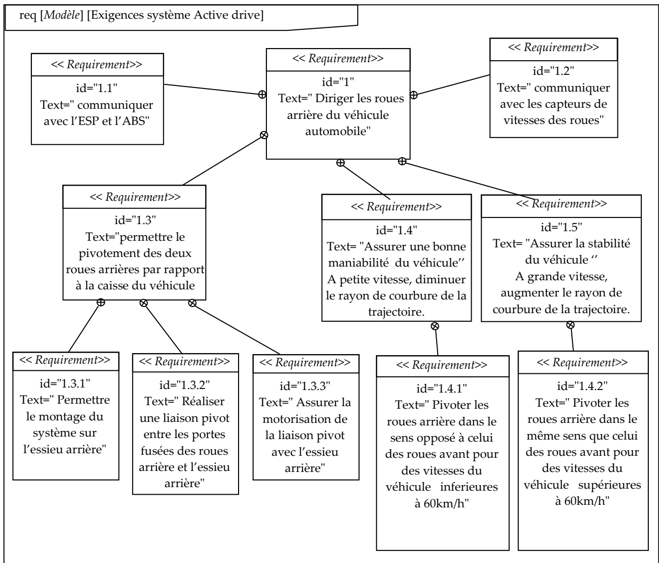
Diagramme des exigences du système 4Control
