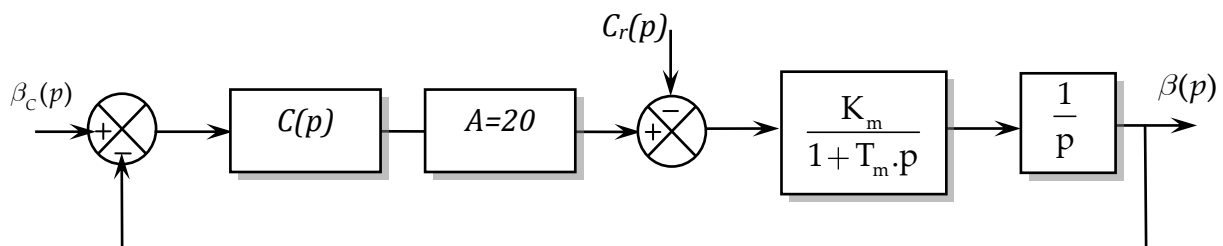
Figure 13 : schéma fonctionnel à retour unitaire
