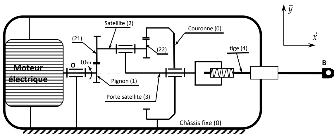
Figure 7 : schéma cinématique du vérin
