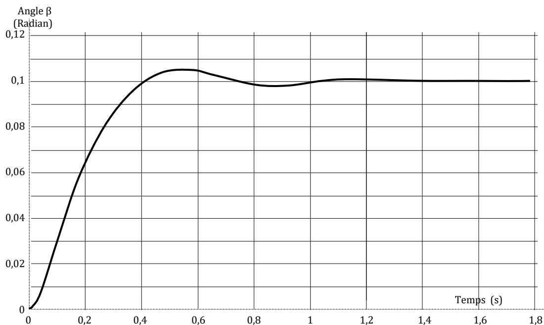
Figure 16 : Réponse indicielle pour la valeur de K_c déterminée à la question 6-18.
